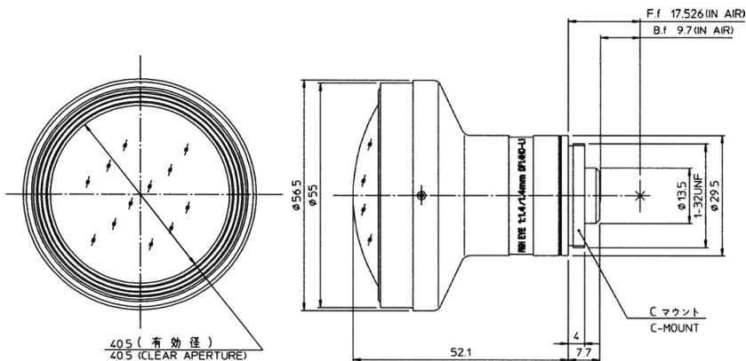
レンズ本体：外観図 Outline drawing DF1.4HC-L1
